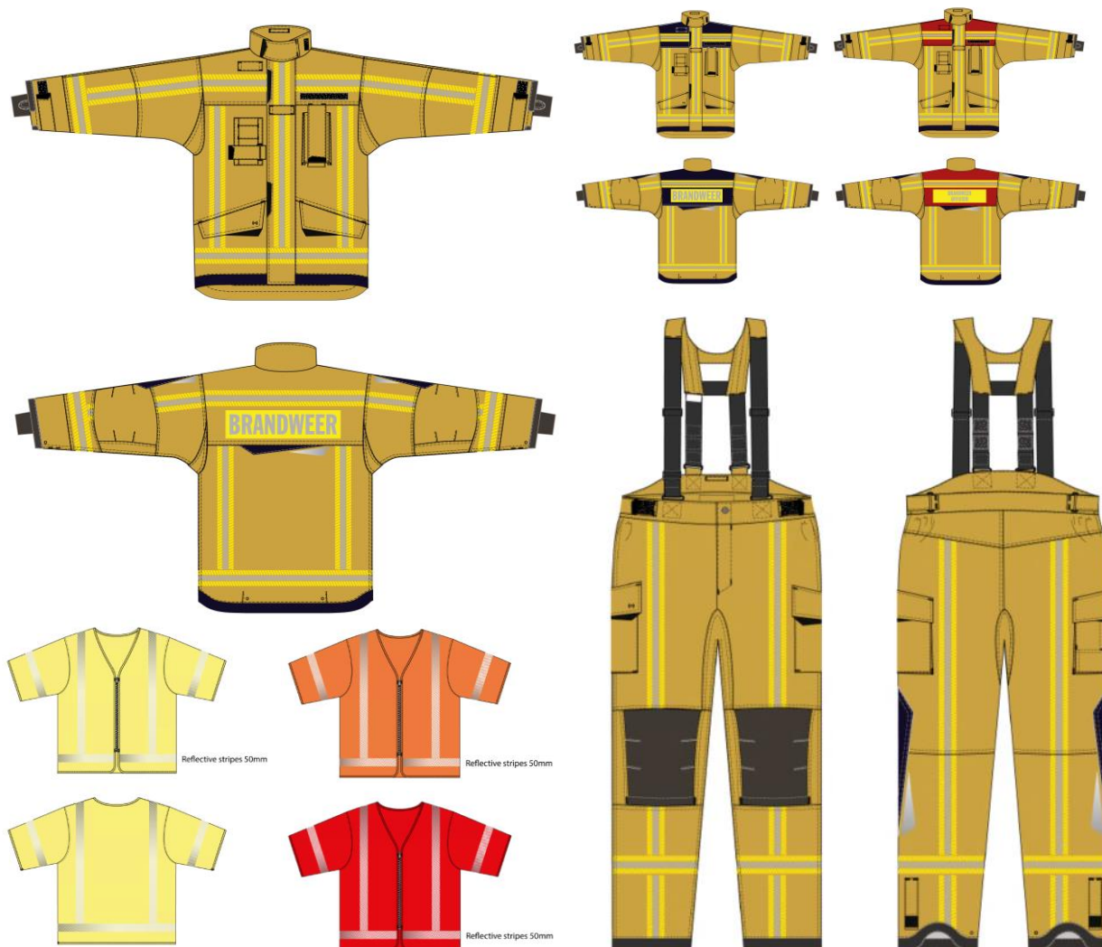
Figuur: Technische tekeningen interventiekledij
